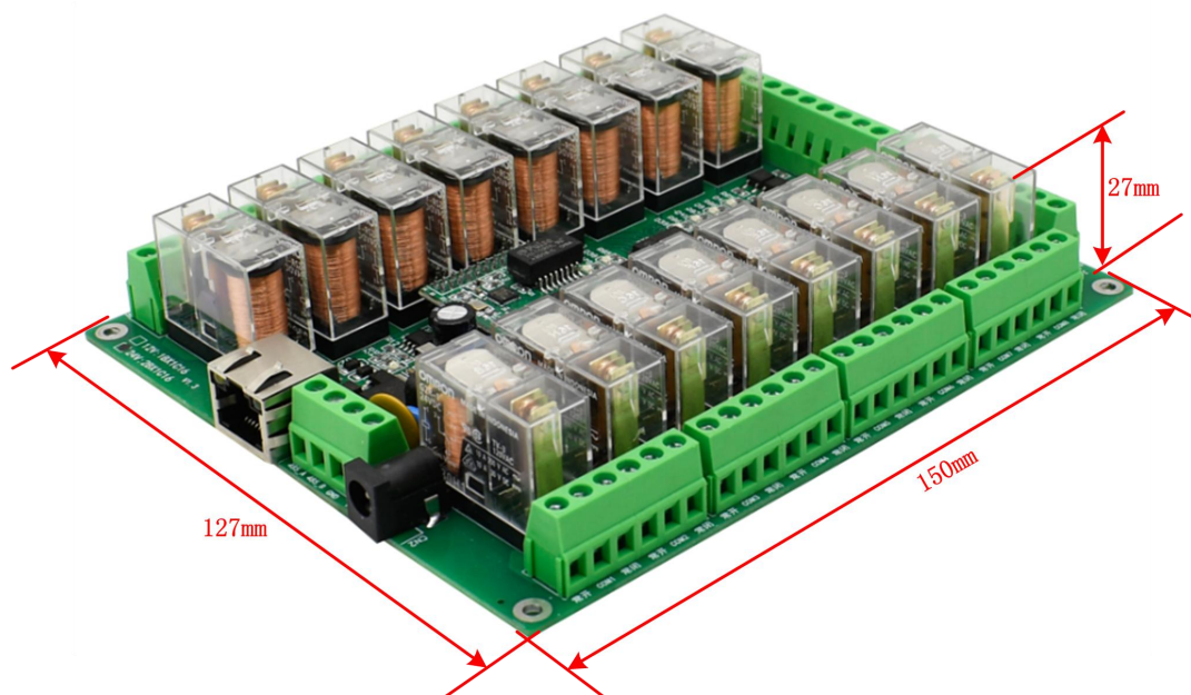
图 4.2 设备机械尺寸 1
