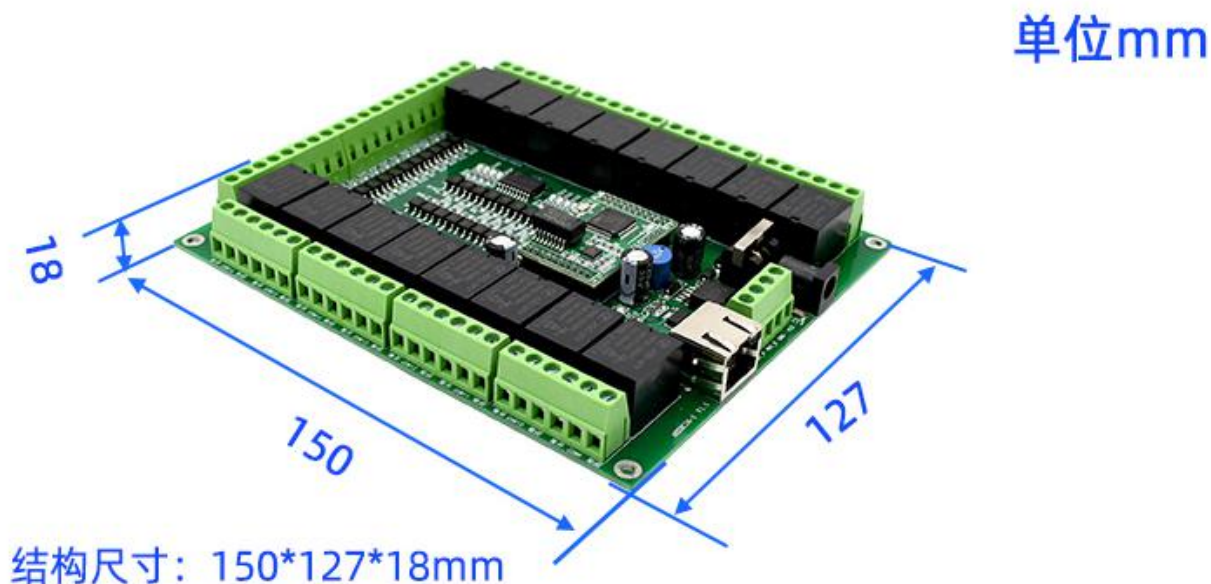
图 4.4 设备机械尺寸 2
