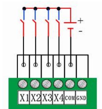
图 4.12 湿节点接法
